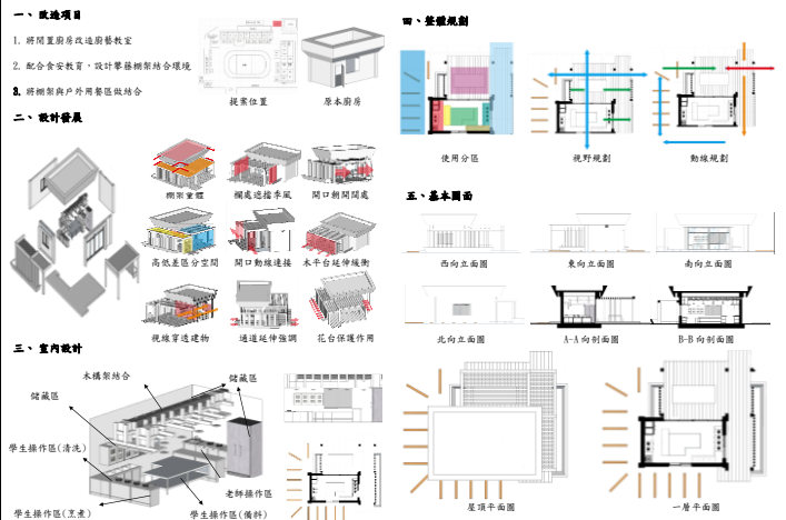
龍坑國小設計圖
